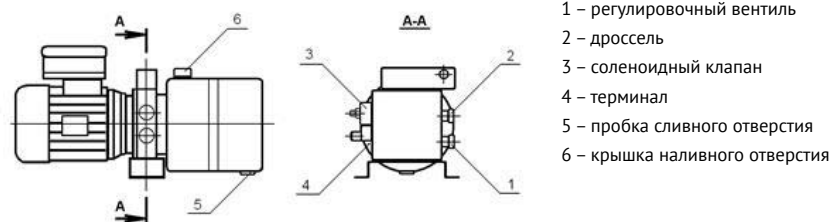
Рис. 8. Гидроузел.
