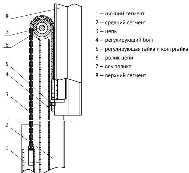
Рис. 9. Трансмиссия.
